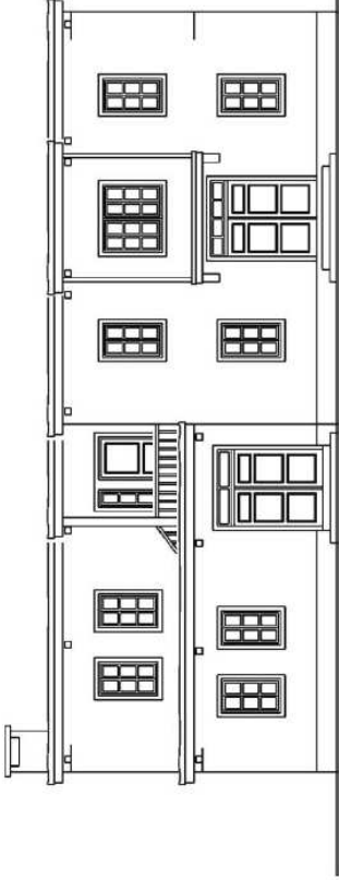
ÖN CEPHE
